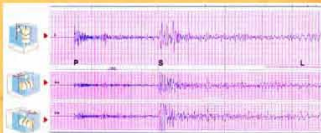
Onde P, L, S, in sismogramma del terremoto in Messico del 20.08.1973 (Osservatorio di Parigi).
